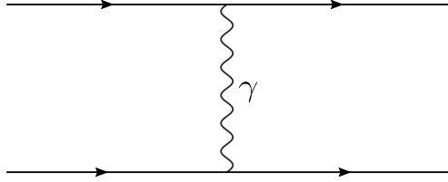
Рис. 1. Пример виртуальной частицы в диаграмме Фейнмана.
