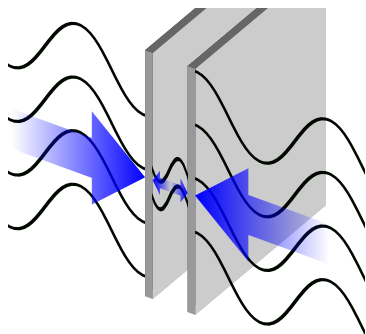
Рис. 7. Силы Казимира, действующие на идеально проводящие пластины.
