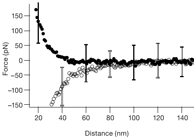
Рис. 8. Заполненные (пустые) кружки показывают силу между золотой сферой и пластинкой из диоксида кремния (золота) в бромбензоле.
