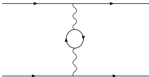
Рис. 2. Превращение виртуального фотона в электрон-позитронную пару.
