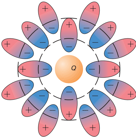
Рис. 1. Экранировка исходного заряда Q поляризованными вакуумными диполями
